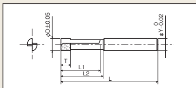
形状 Dimensions
