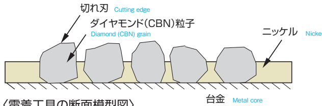
〈電着工具の断面模型図〉
