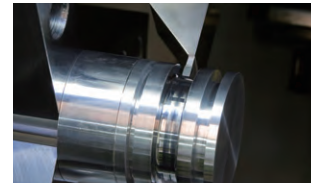
アルミ合金の旋盤加工 Lathe processing of aluminum
