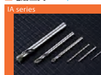
[20ページ] (page 20) 電着ドリル ドリルタイプ (スパイラル形状) Electroplated drill type (spiral flute)
