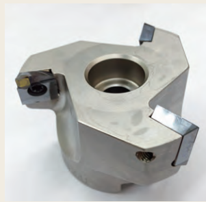
単結晶ダイヤモンドカッター Single-diamond cutter
