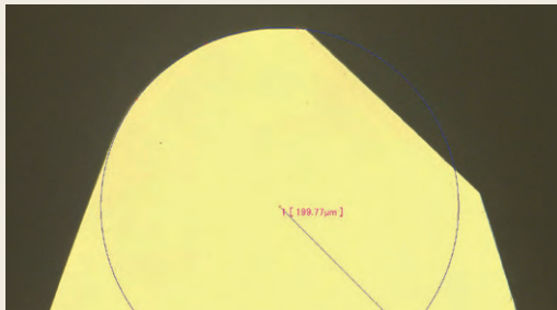
ミュラーエンドミルボール TYPE-II 刃先 The edge of Muller End Mill Ball type-II
