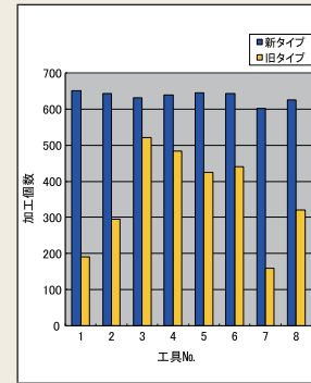
電着ドリルライフテスト (当社比) Electroplating Drill Life Test (EISEN comparisons)
