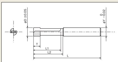
形状 Dimensions
