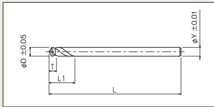
形状 Dimensions
