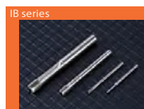
[20ページ] (page 20) 電着ドリル フラットタイプ (直刃形状) Electroplated drill flat type (straight flute)
