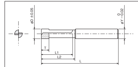
形状 Dimensions
