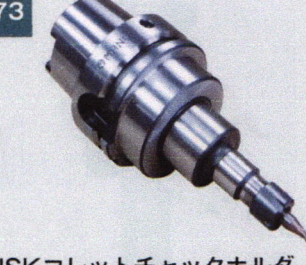
HSKコレットチャックホルダ HSK COLLET CHUCK HOLDER
